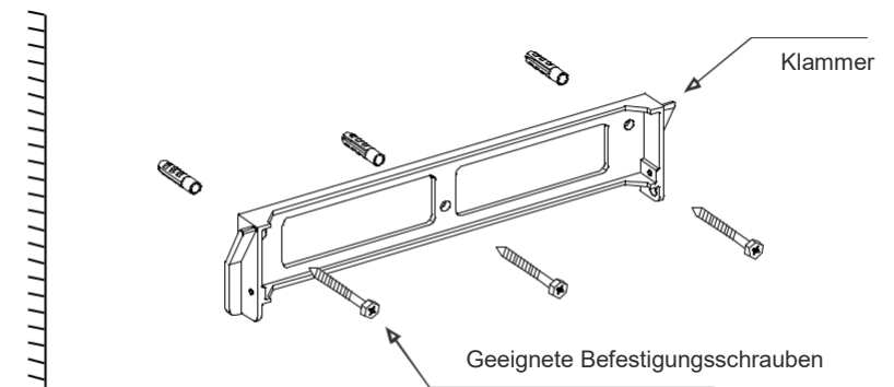
Abbildung 4.4 Wechselrichter-Wandmontage
