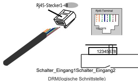
Abbildung 4.28 Abisolieren der Isolierungsschicht und Anschluss an RJ45-Stecker
