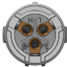
Abbildung 4.13 AC-Netzanschlusstecker innen
