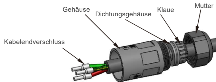
Abbildung 4.14 AC-Netzanschlussklemme
