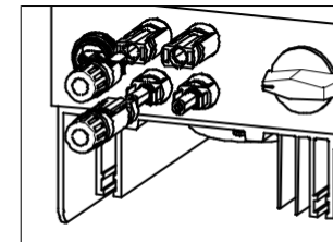
Abbildung 4.12 Anschluss der DC-Anschlüsse an den Wechselrichter
