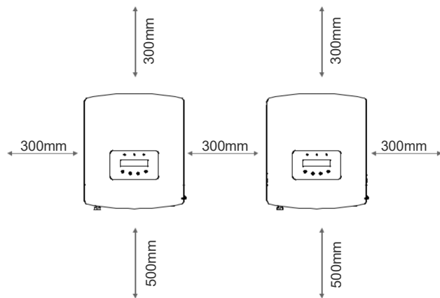
Abbildung 4.2 Montageabstand des Umrichters
