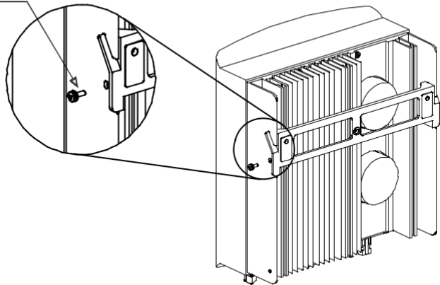
Abbildung 4.5 Wandhalterung
